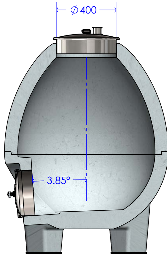
SECTION A-A SCALE 1 : 16
